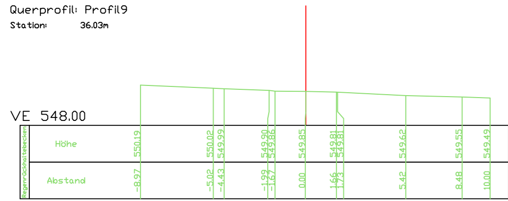
Längsprofil_1 HNN+545.57
